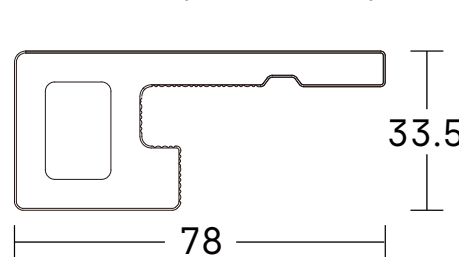
INNER CORNER (VERTICAL)-HLYC-020F
